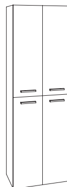
HTT6 Breite 60,0 cm Höhe 178,7 cm Tiefe 34,8 cm
